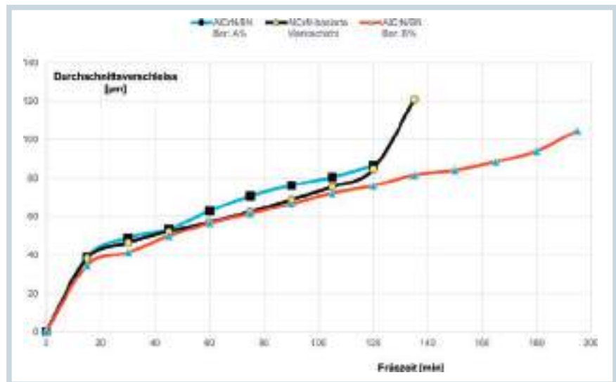
3 Standzeitvergleich beim Taschenfräsen mit Schafffräsern bei Variation des BN-Anteils per Software. Fräsen mit vierzahnigem 8-mm-Fraisa NX-V Torus in 1.2085 (HRC 29,2), a_p = 5 \text{ mm} , a_e = 5,5 \text{ mm} , v_c = 120 \text{ m/min} , f_z = 0,06 \text{ mm/Z} , MMS, Durchschnittsverschleiß (maximaler Rundfasenverschleiß + VB_{max} + Stirnverschleiß + Eckverschleiß) / 4 (© Platit)
