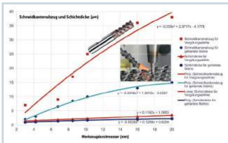
6 Typische Voreinstellparameter beim Beschichten von VHM-Schaftfräsern (© Platit)
