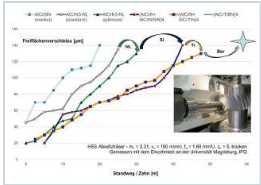
5 Einfluss der Materialkomponenten in den Schichten am Beispiel eines HSS-Wälzfräasers ( m_n = 2,31 ; v_c = 10 m/min; f_a = 1,69 mm/U; z_o = 5 , trocken); gemessen mit dem Einzahnstest an der TU Magdeburg. Alu macht hitzefest, Chrom zäh und verschleißfest (abrasiv); Al/Cr/Ti-Nanolayer steigern die Zähigkeit, Titan minimiert Ausbrüche, und Bor erhöht die chemische Stabilität (© Platit)
