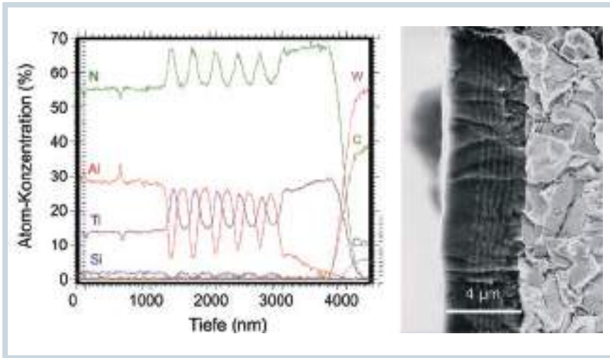
2 Struktur einer sogenannten Triple-Schicht. Von innen nach außen beginnt es mit Titanitrid (TiN) oder Chromitrid (CrN), dann folgt der mittlere Abschnitt als extrem zähe, mehrlagige Struktur, und es folgt eine sehr harte Deckschicht (© Platit)
